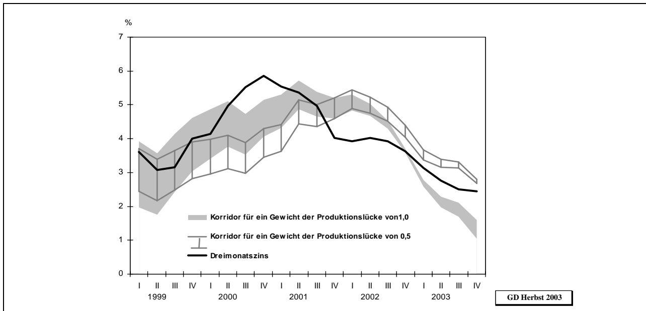
Abbildung 5.1: Taylor-Regeln für den Euroraum
